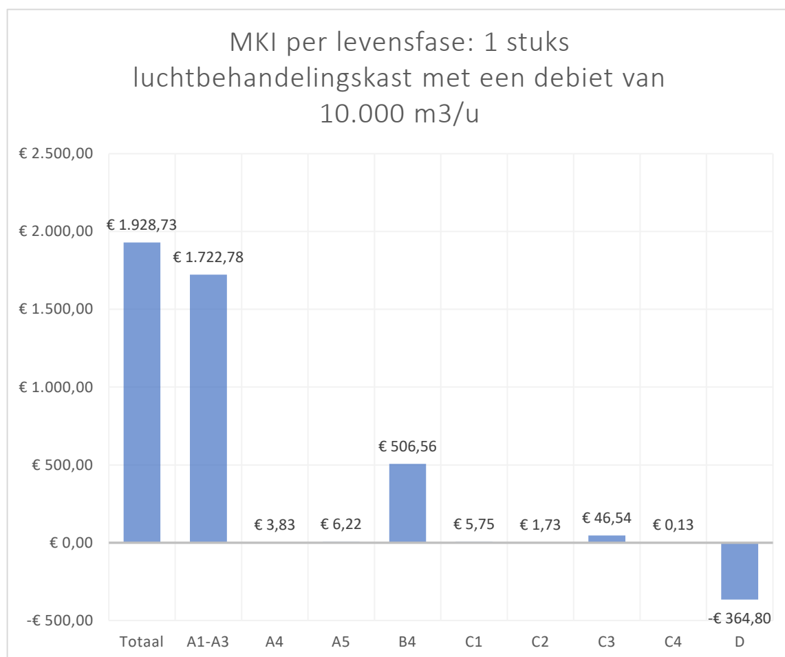
Figuur 9 - Impact per levenscyclusanalyse luchtbehandelingskast
